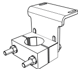
900234000Q0030 #2 Motor bracket x1
